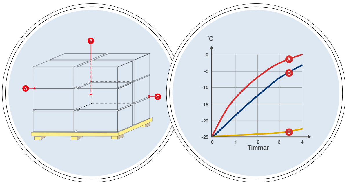
BILD 3: TEMPERATURHÖJNING I EN LASTPALL MED FRYST STUVAD SPENAT VID EN OMGIVANDE LUFTTEMPERATUR PÅ +15°C
